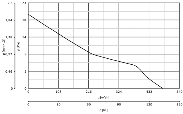
VORTICE 230/9" ARI cod 12453
