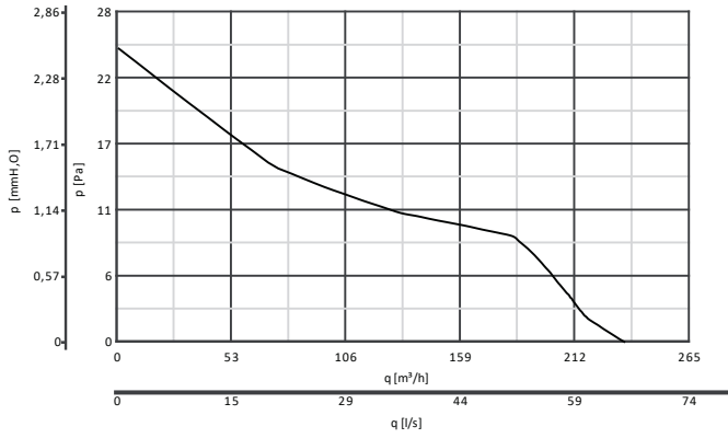
VORTICE 150/6" ARI cod 12613
